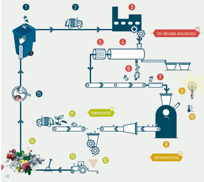
Le cycle de valorisation à l'usine de tri-méthanisation-compostage Ovade
